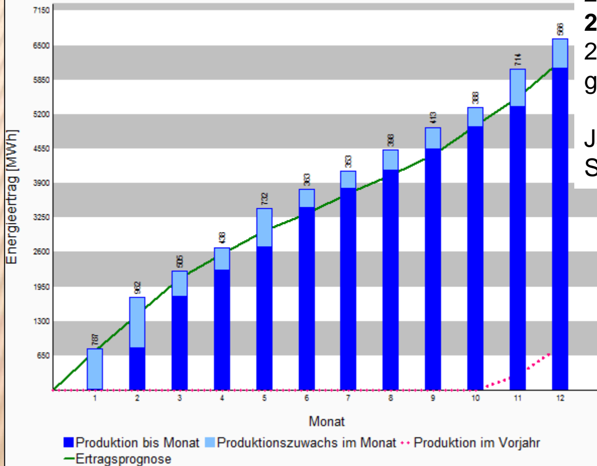
Stromproduktion Kammerberg - 1150175 2016 kumuliert
